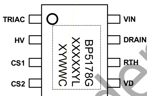
图2 管脚封装图
